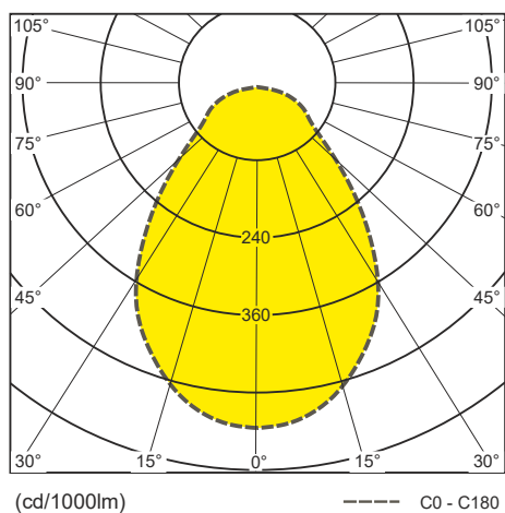
Bryła fotometryczna
